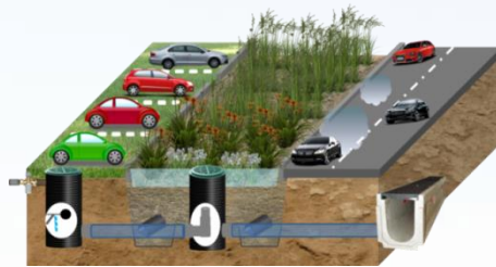
道路邊灌溉型RGD-雨水花園 Bioretention
