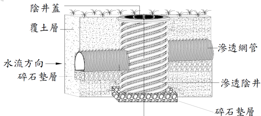
DMW-滲透陰井參考圖
